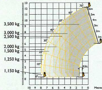
535-125 HiViz Stabilisers extended
