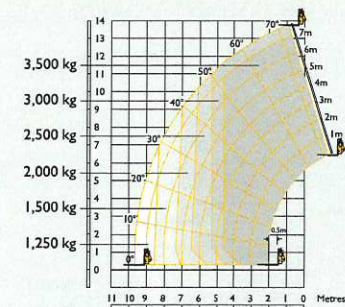
535-140 HiViz Stabilisers extended
