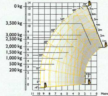
535-140 HiViz Stabilisers retracted
