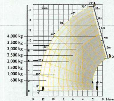
540-170 Stabilisers extended
